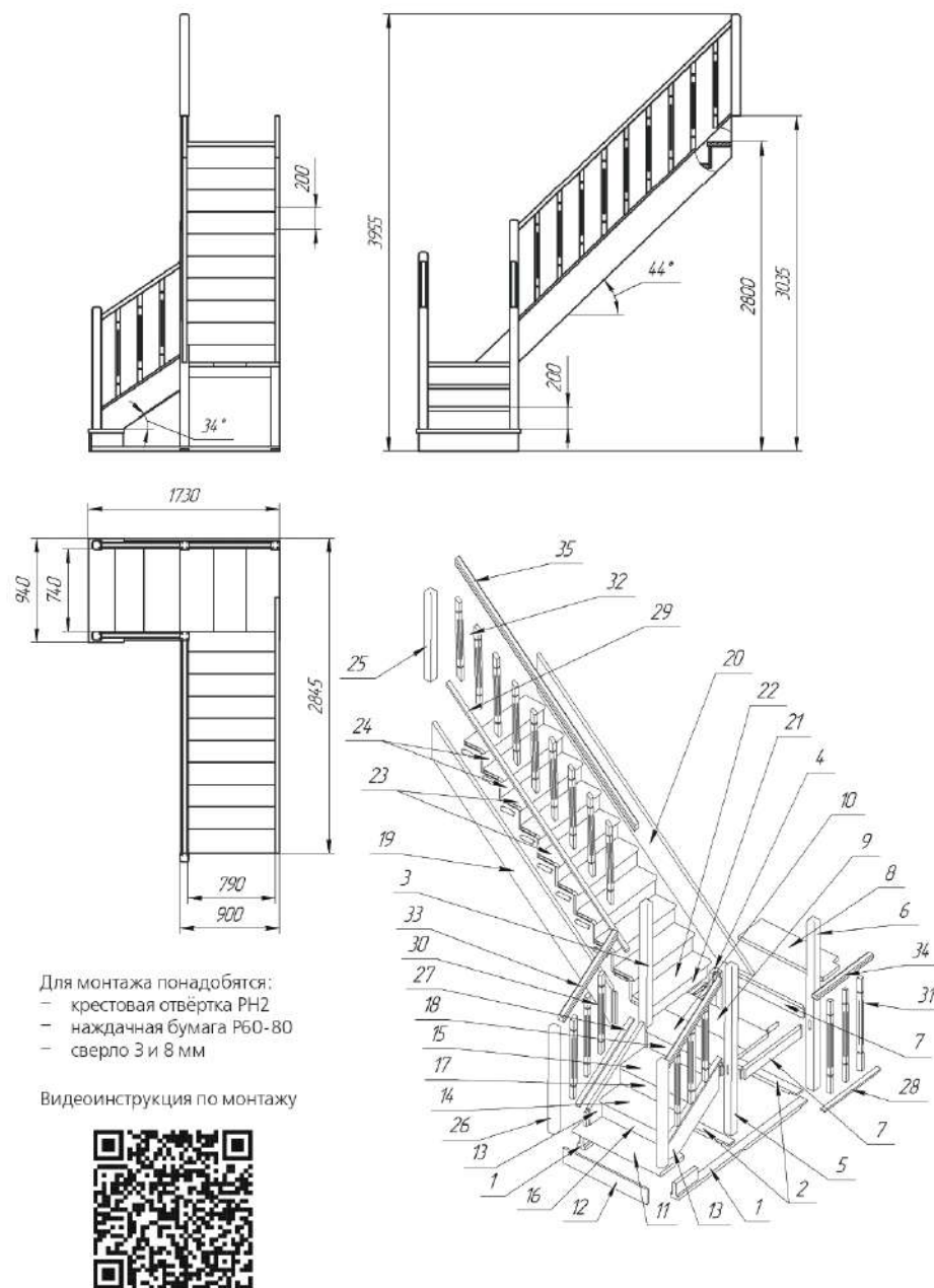
Рисунок 1. Лестница внутриквартирная ЛЕС-04.
